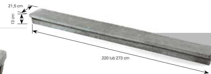
Belka podwalinowa (zbrojona) symbol: D3 (220 cm) waga: ok. 80 kg symbol: D3 (273 cm) waga: ok. 95 kg
