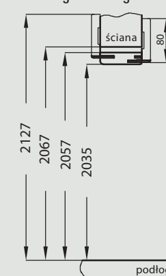
Przekrój pionowy tunelu regulowanego TOP
