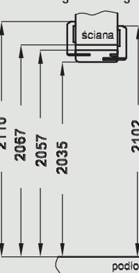
Przekrój pionowy tunelu regulowanego
