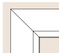
SPOSÓB ŁĄCZENIA OPASEK SYSTEM DUO (80 mm)
