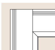
SPOSÓB ŁĄCZENIA OPASEK SYSTEM NOBLE – WERSJA A (100 mm)
