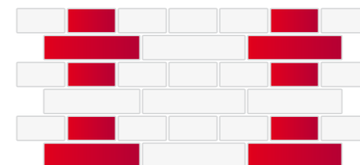
WIĄZANIE KRZYŻOWE TYP 1
