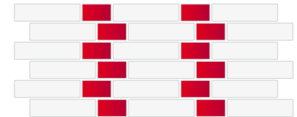
WIĄZANIE GOTYCKIE
