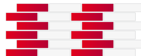
WIĄZANIE WOZÓWKOWE PRZESUNIĘCIE 0 1/3 CEGŁY
