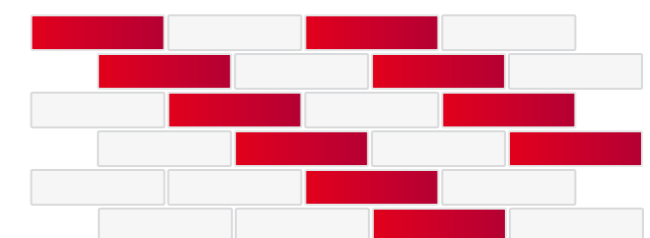
WIĄZANIE WOZÓWKOWE PRZESUNIĘCIE 0 1/4 CEGŁY
