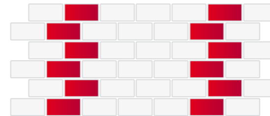
WIĄZANIE GŁÓWKOWE
