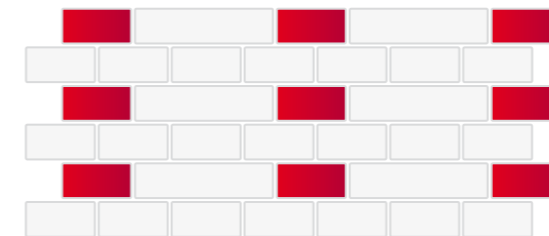
WIĄZANIE HOLENDERSKIE
